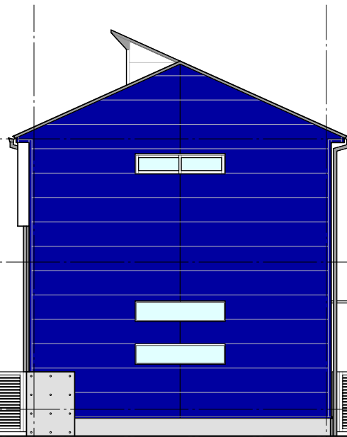
東立面図 S=1/100
