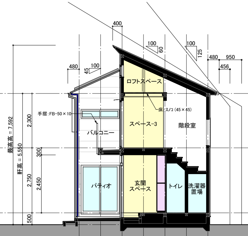
断面図 S=1/100
