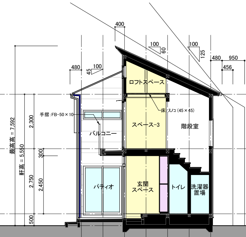
断面図 S=1/100
