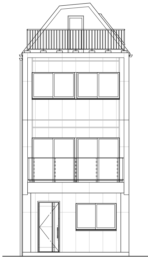
南 (道路側) 立面図 S=1/100
