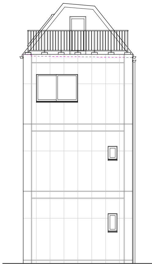
北立面図 S=1/100
