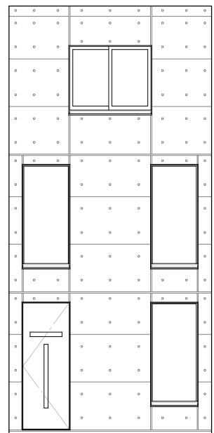
道路側立面図 S=1/100
