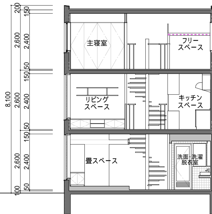
断面図 S=1/100
