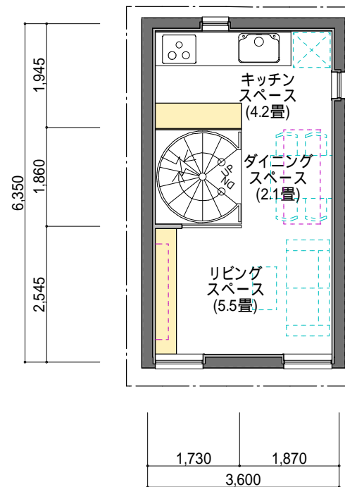
2階平面図 S=1/100
