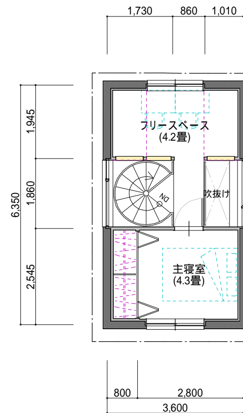
3階平面図 S=1/100
