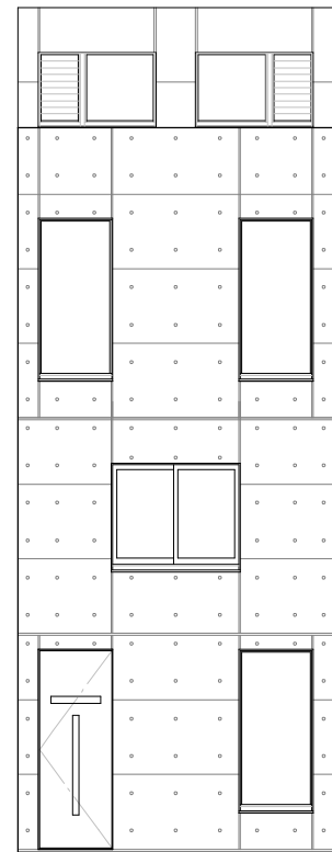
道路側立面図 S=1/100
