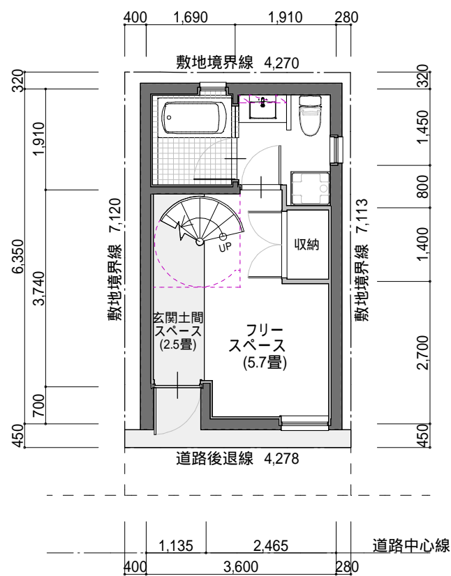
配置・1階平面図 S=1/100
