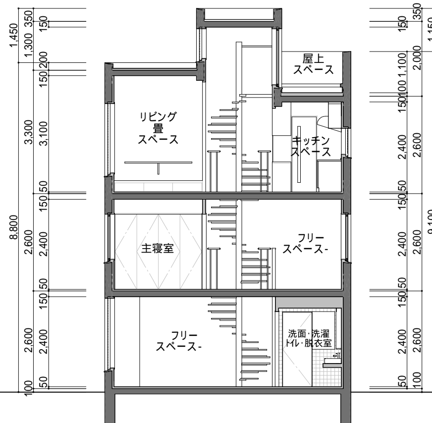
断面図 S=1/100
